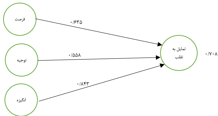
شکل ۳- آماره t-value الگوی کلی پژوهش با روش بوت استراپ
