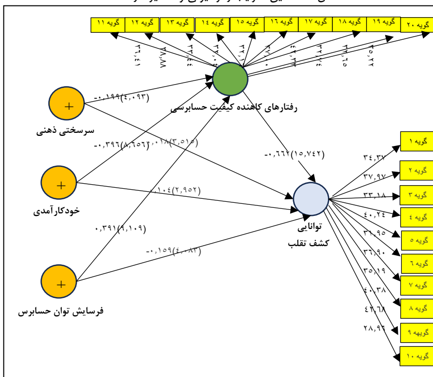
شکل ۱- تخمین ضرایب رگرسیونی و مقادیر آماره t
